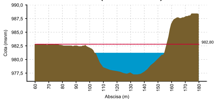
CAUCA - LA BALSA (28/06/2021 06:00 AM) NIVEL= 981.18
